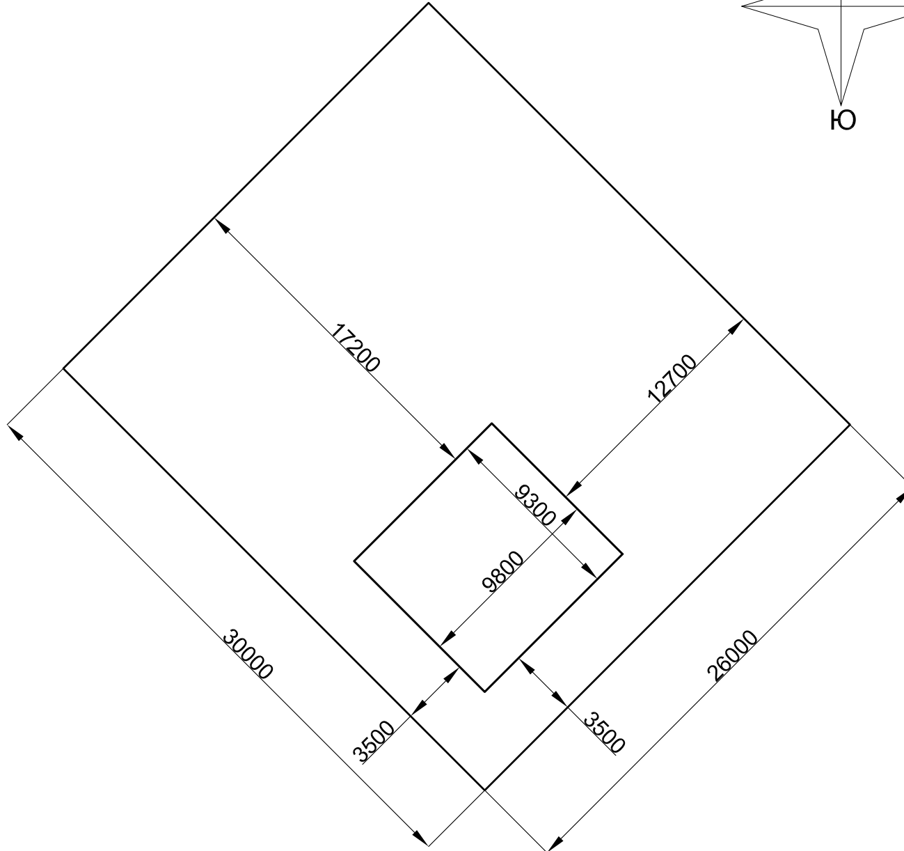
Схема планировочной организации земельного участка
